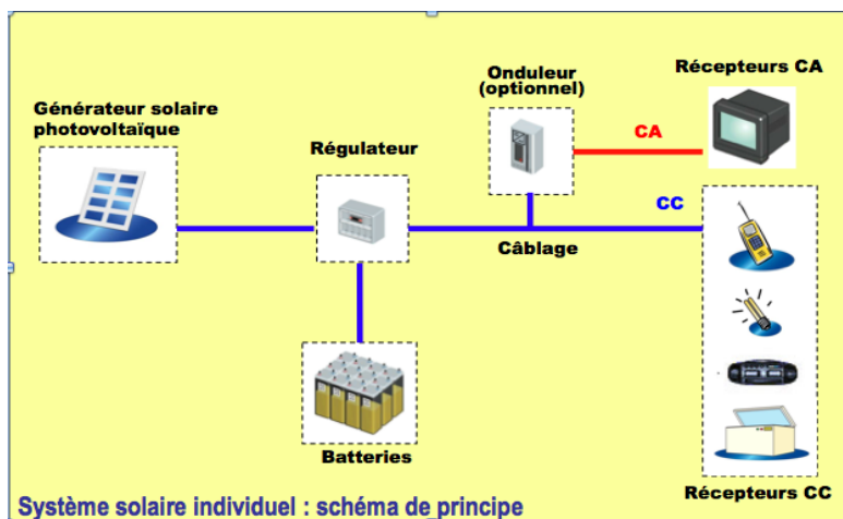
Figure1 : un kit solaire photovoltaïque individuel
